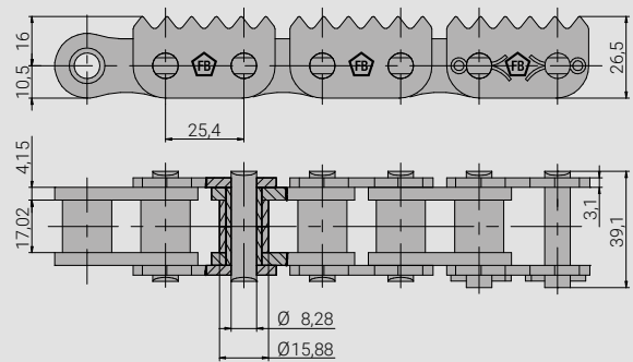
16B-1FBVERZAHNT6x50,8
