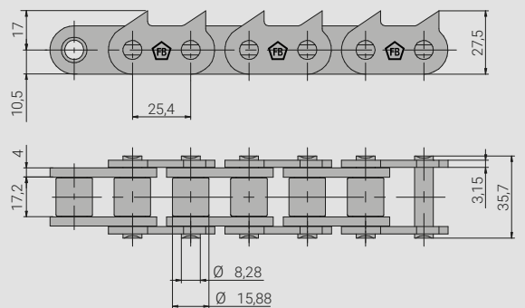
16B-1FBSÄGEVERZ2x50 5118.000.51
