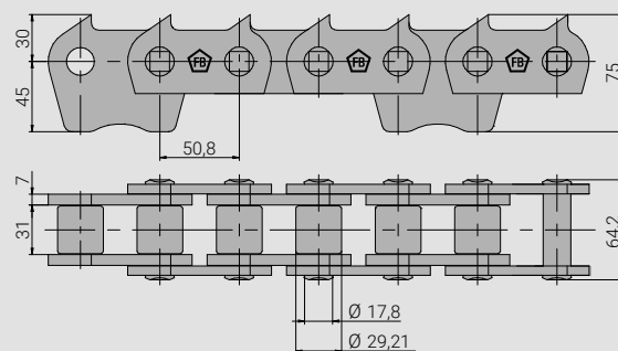
32B-1FBVERZS2/PLx203,2I
