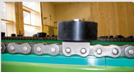
Bretterquerförderer
