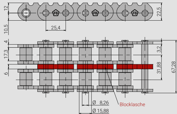
16B-2TFVERZ3x25,4
