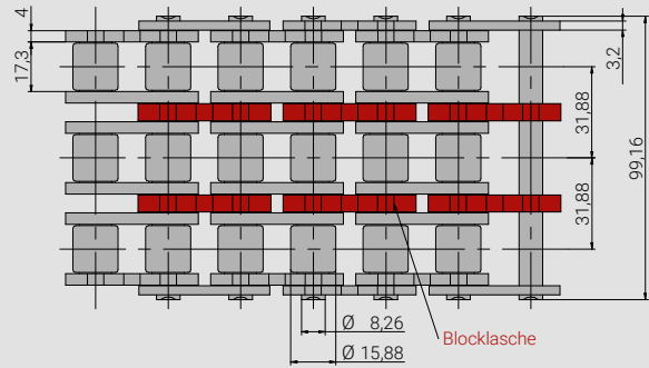
16B-3FBFVERZ/PLx101,6
