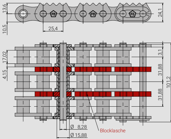
16B-3FBVERZ5H24
