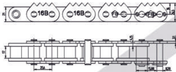
16B-1FBVERZAHNTx50,8 / 5118.000.34
