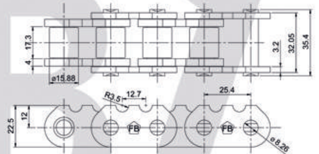
16B-1FVERZ93020505
