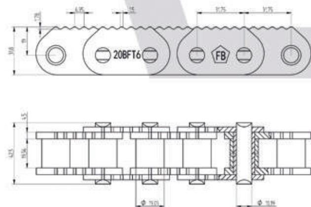
5130.000.23FB
