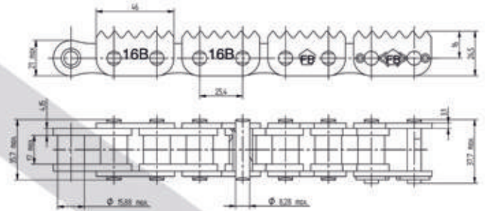
16B-1FBVERZAHNT6x50,8
