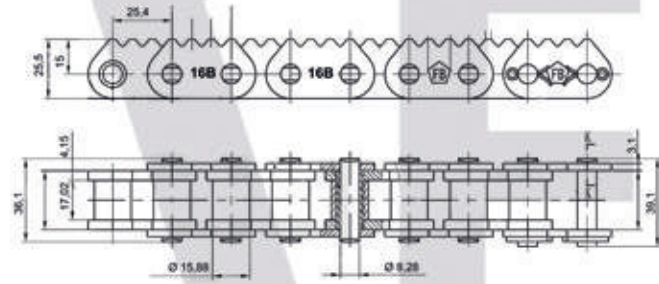
5118.000.35 / ISO 16B-1
