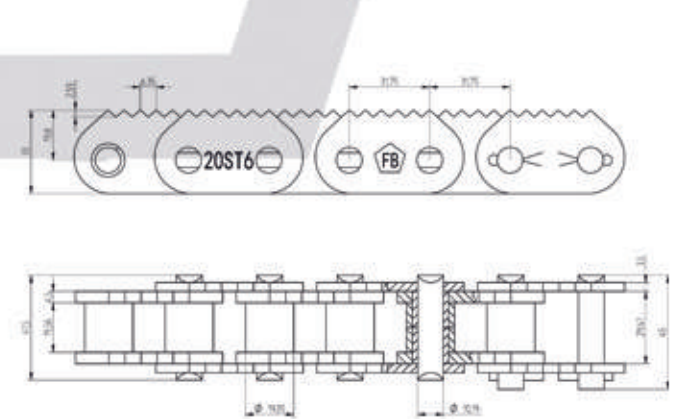
5130.000.22FB
