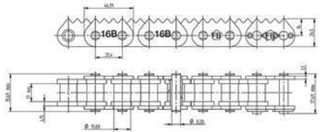
16B-1FBVERZAHNT
